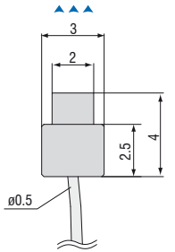
cable length 0.25 m ± 0.04 m
