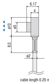
cable length 0.25 m
