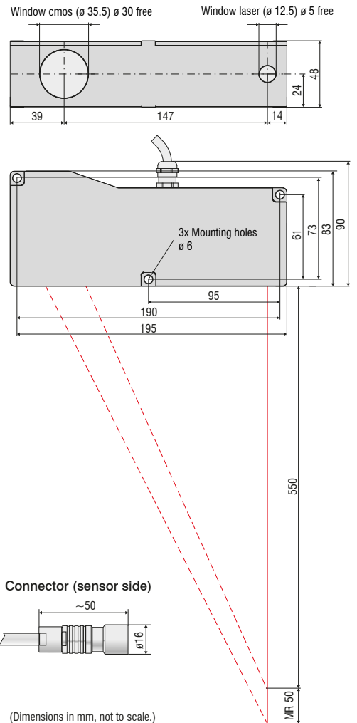
optoNCDT 2310-50
