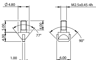
1 x 6 mm Blade Edge
