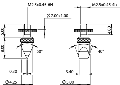
Knife Edge
