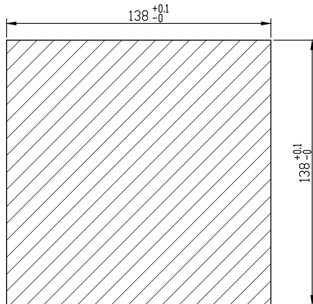
パネルカット寸法 Panel Cut Dimension
