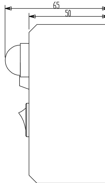
PW-01 外形图 OutLine Drawing
